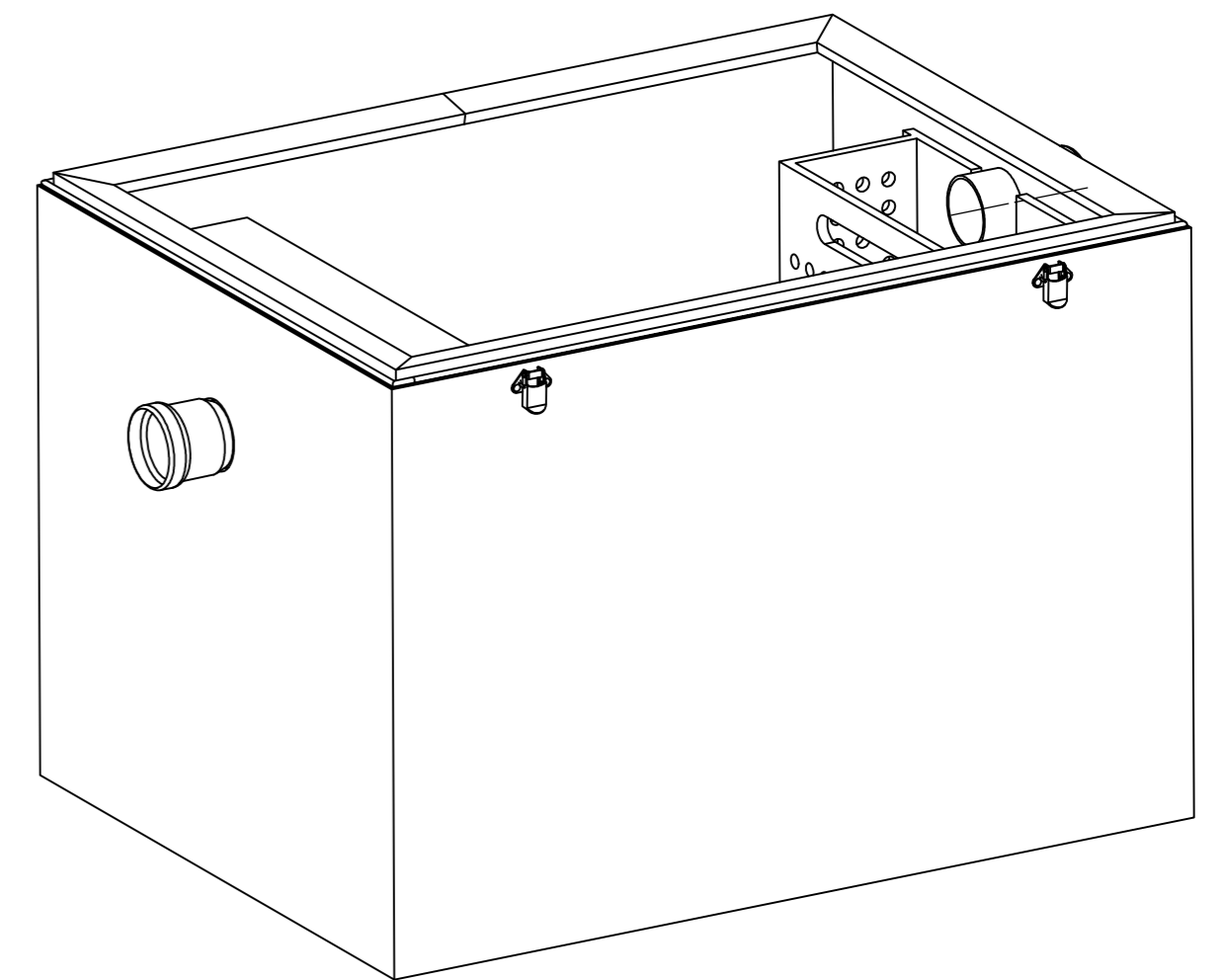
3D Вид 3
